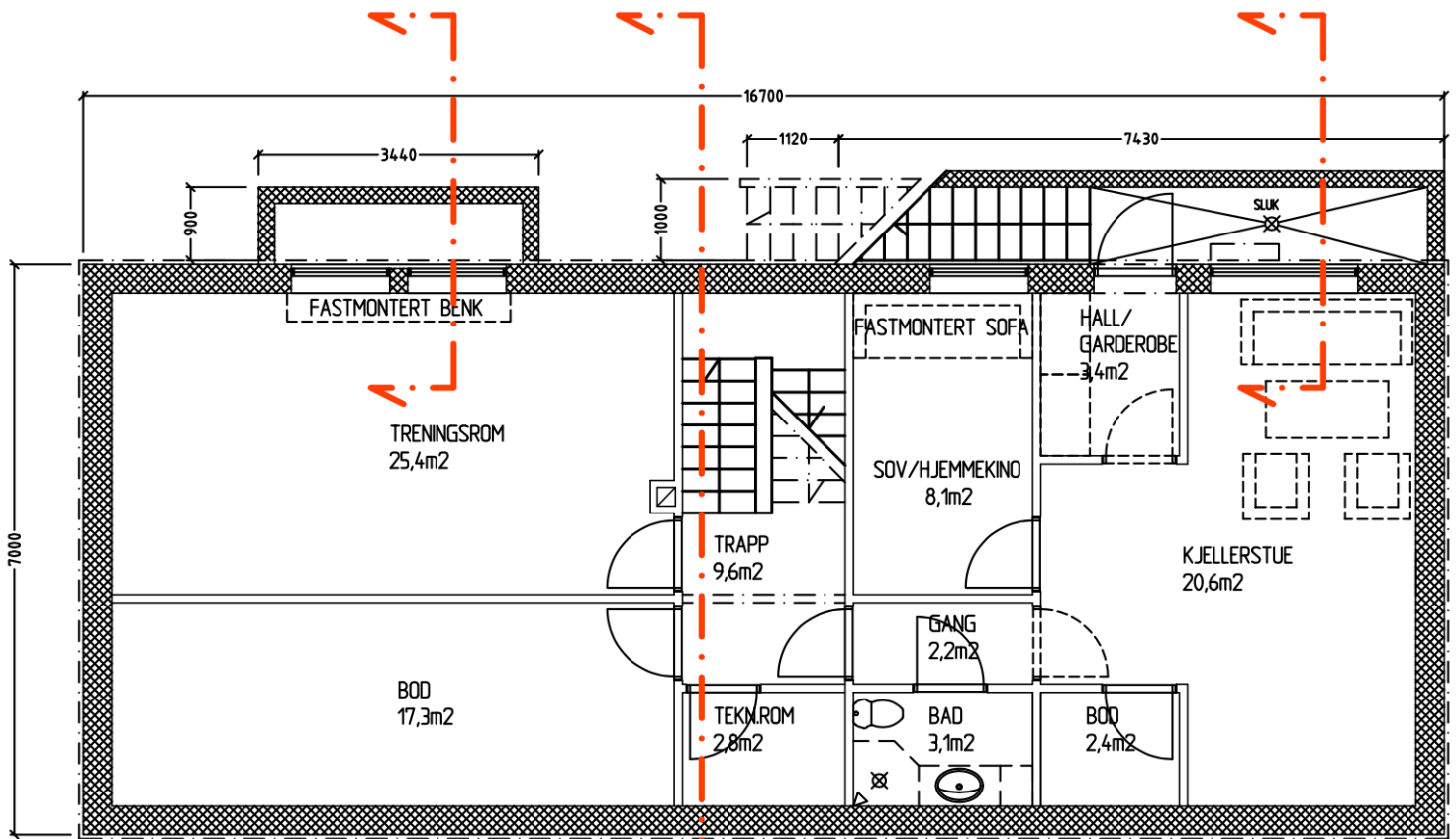
PLAN KJELLER
