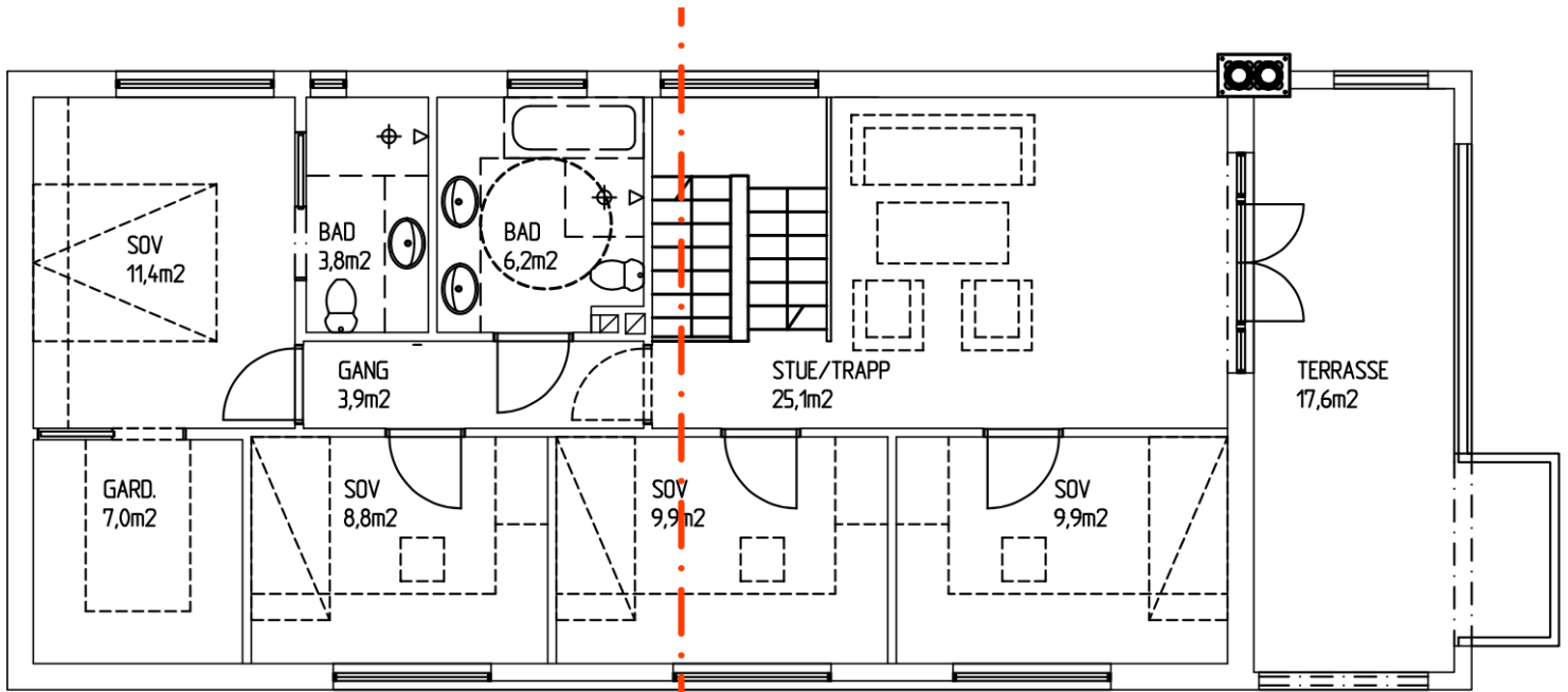
PLAN 2. ETASJE
