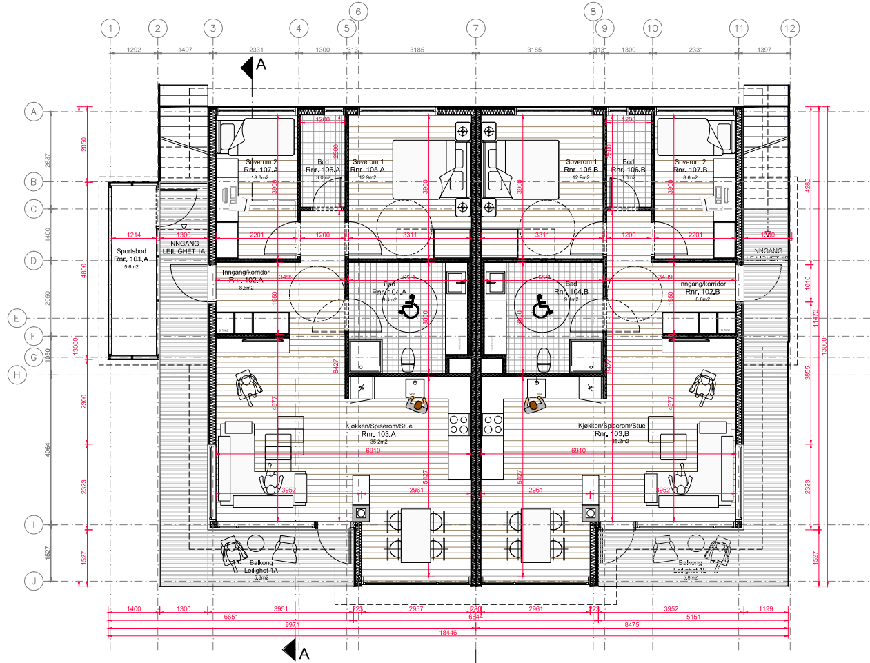
PLANLØSNING 1ETG. 1:100
