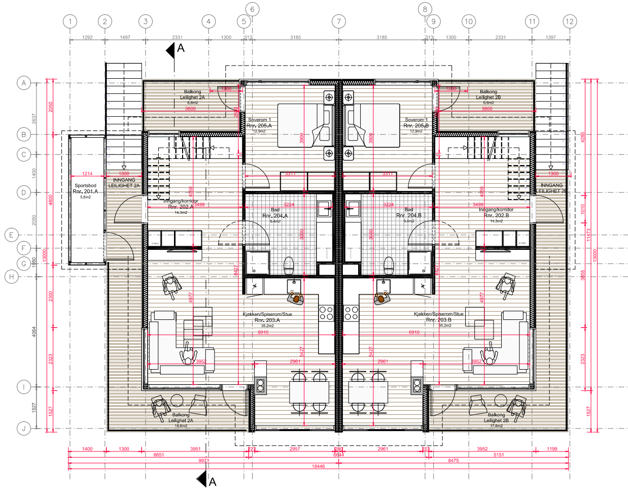
PLANLØSNING 2ETG. 1:100
