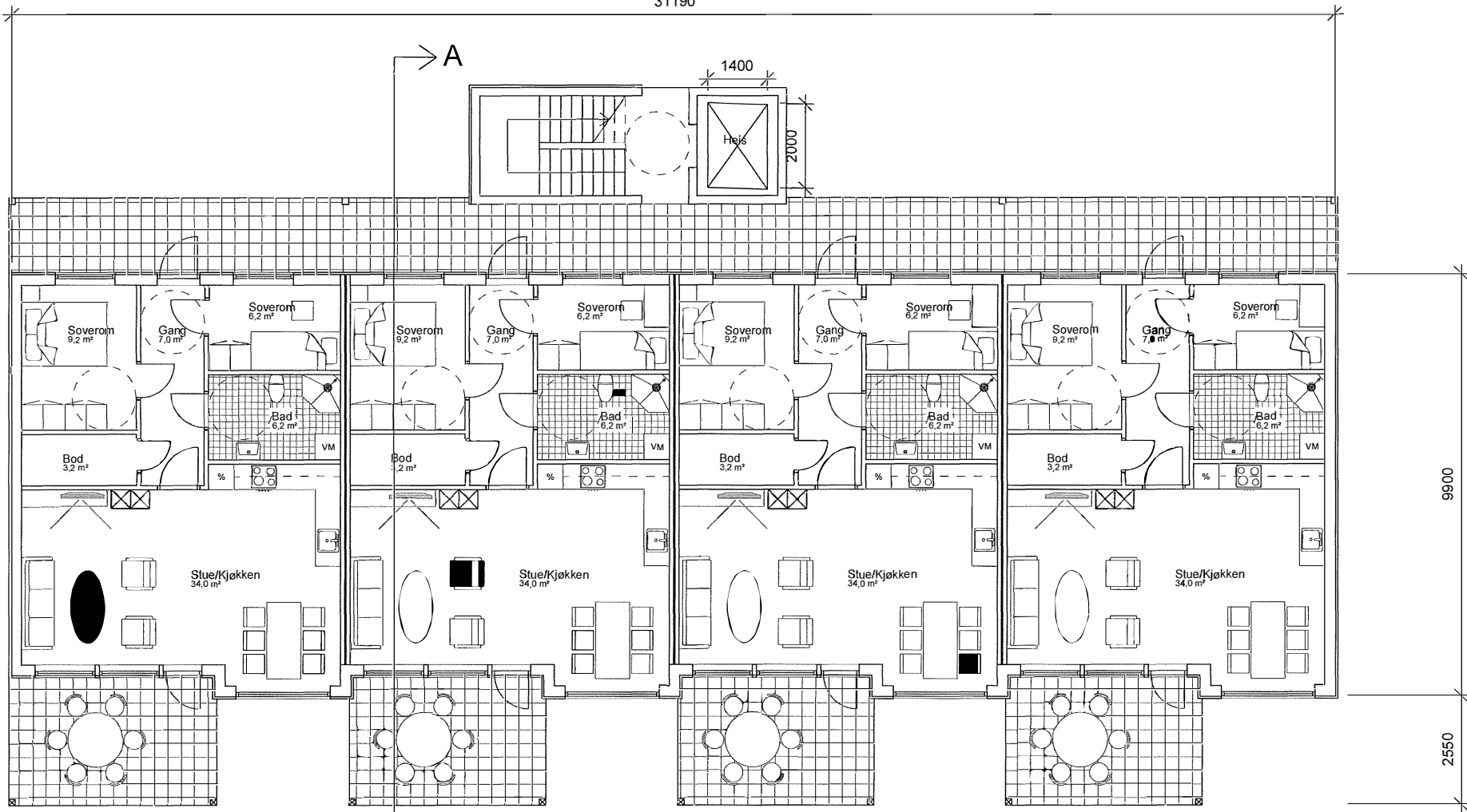
PLAN 1.ETG
